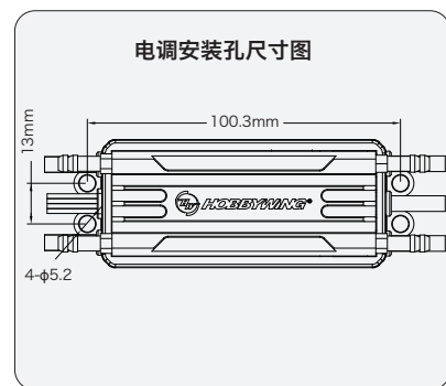
SEAKING 160A V4
